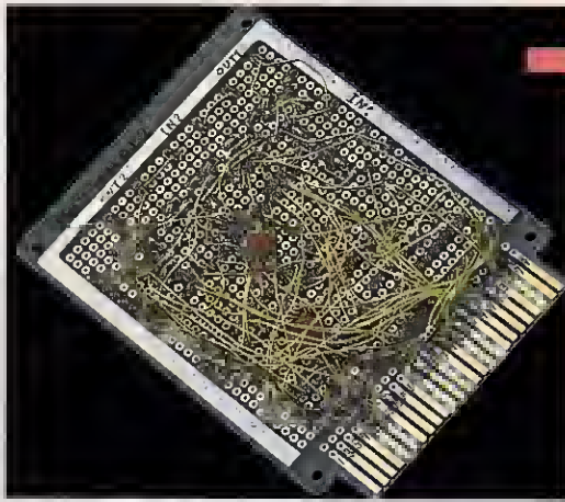
◆これが裏面だ。狭くて表に取り付けられなかった部品が見える。こんな風に臨機応変にやるといいね。
